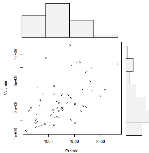
Slika 2: Razsevni graf pretokov [m 3 /s] in volumnov [m 3 ] visokovodnih valov Save v Litiji (1953-2010).
