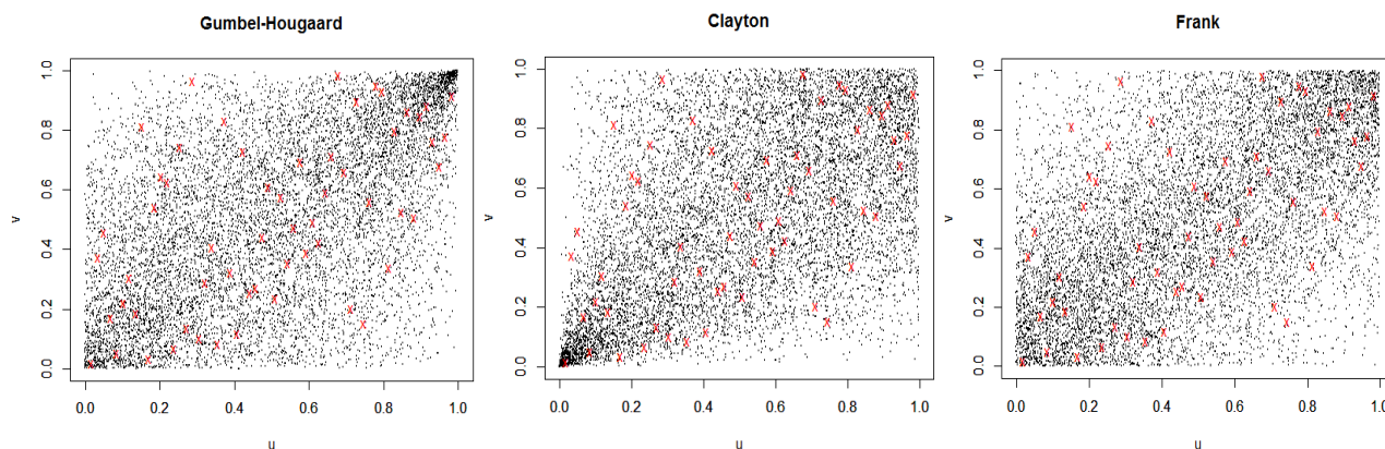
Slika 3: Prikaz ujemanja med generiranimi in izmerjenimi podatki za tri teoretične funkcije kopula.
