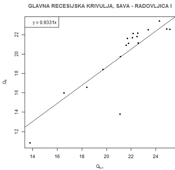
Slika 7: Primer glavne recesijske krivulje ( k = 0,933 ) (vodomerna postaja Radovljica I).
