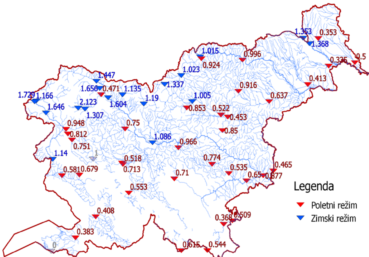
Slika 8: Razmerje sezonskosti RS za obravnavane vodomerne postaje v Sloveniji.
