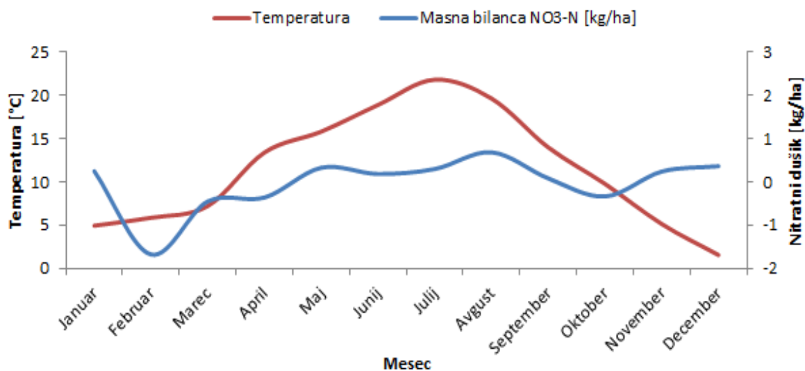
Slika 10: Povprečne mesečne temperature zraka in mesečne bilance nitratnega dušika v letu 2007.
