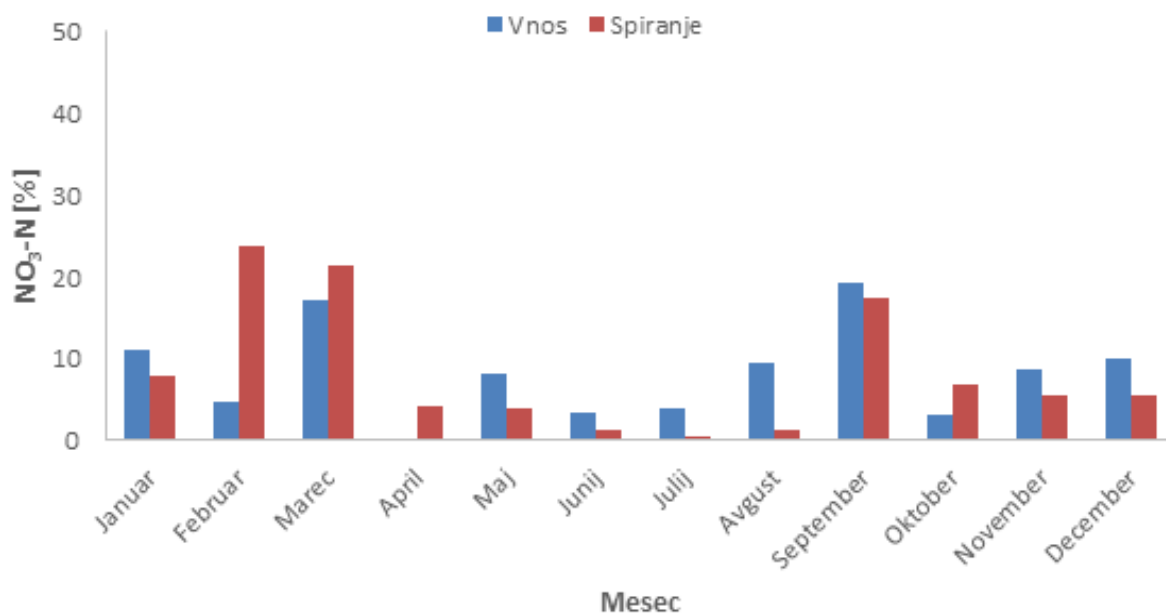
Slika 8: Mesečni deleži masne bilance atmosfersko vnesenega in spranega nitratnega dušika na porečju Padeža glede na letne količine, leto 2007.
