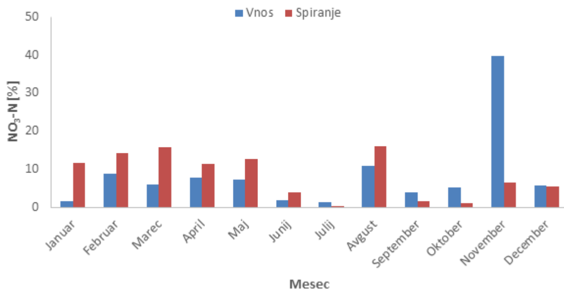
Slika 7: Mesečni deleži masne bilance atmosfersko vnesenega in spranega nitratnega dušika na porečju Padeža glede na letne količine, leto 2006.
